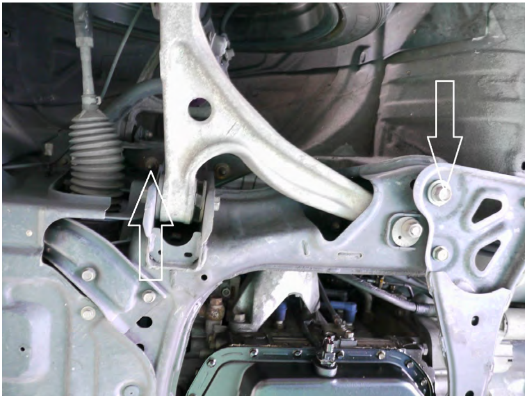
フロント
